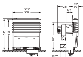
Einbauabmessungen S 3004
