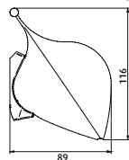
Gehäusemaße (mm)
