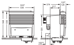
Einbauabmessungen S 5004
